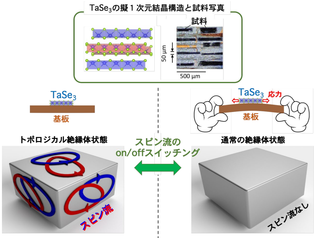
図 1：（上図） TaSe 3 は、鎖状の構造が積み重なって形成されるため、擬一次元的な結晶構造と電気伝導を示す。（左下図）外から歪みを加えない状態の TaSe 3 はトポロジカル絶縁体状態となり、結晶の表面にスピンの流れが生成されることが分かった。（右下図）基板に試料を乗せ、それをたわませると、赤い矢印方向に応力が印加され試料に歪みが生じる。その結果、TaSe 3 は通常の絶縁体となりスピンの流れが消失する。基板をたわませる・たわませないの簡単な操作で、スピンの流れの on/off スイッチングが可能となる。
