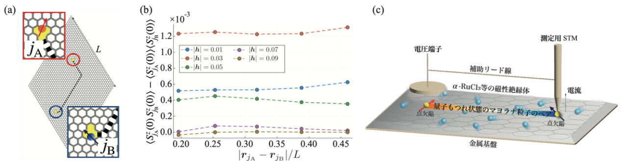
図 2. (a) 今回の研究で取り扱った理論モデル。遠く離れた 2 地点に点欠陥が導入され、量子もつれ状態を形成するマヨラナ粒子がそれぞれに束縛されている。点欠陥に隣接したスピンサイトを j_A , j_B と名付ける。 L はシステムの大きさ。(b) 量子テレポーテーション現象のシミュレーション結果。横軸は導入される点欠陥間の相対距離、縦軸は量子テレポーテーション現象の大きさ(非局所スピン相関)を表す。相対距離が大きくなっても非局所スピン相関は単調に減少することなく、ほぼ一定の値を取り続けることが確認できる。 |h| は外部磁場の大きさ。(c) 量子テレポーテーション現象を測定できる実験セットアップ。点欠陥に束縛されたマヨラナ粒子の量子もつれによって、電気伝導度が有限になる。STM のトンネル電流を利用するため、磁性絶縁体は伝導基盤上に接合する。
