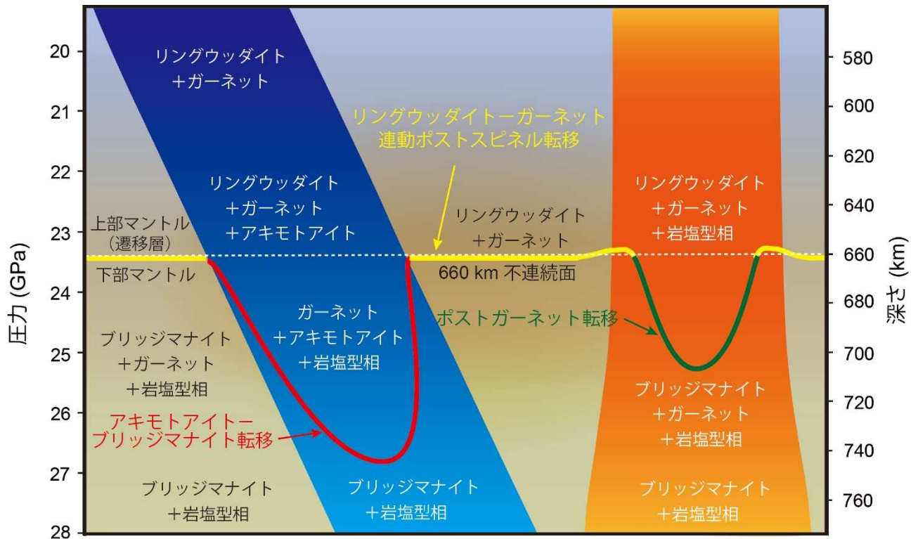
図 1. 地震学的に観測されている地球マントル 660 km 不連続面の凸凹構造。青帯：沈み込んだ低温のプレート（例：トンガ・マリアナ沈み込み帯直下）、オレンジ帯：マントル深部から上昇した高温のプルーム（例：ハワイホットスポット直下）、黄線：リングウッドイトーガーネット連動ポストスピネル相転移による 660 km 不連続面、赤線：アキモトアイトーブリッジマナイト相転移による 660 km 不連続面の陥没、緑線：ガーネットーブリッジマナイト相転移（ポストガーネット転移）による 660 km 不連続面の陥没。
